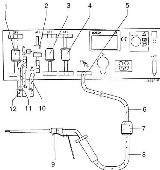
Rys. 1, Schemat połączeń toru pomiarowego na tylnej ścianie analizatora:
